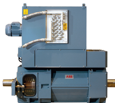
直流电机
