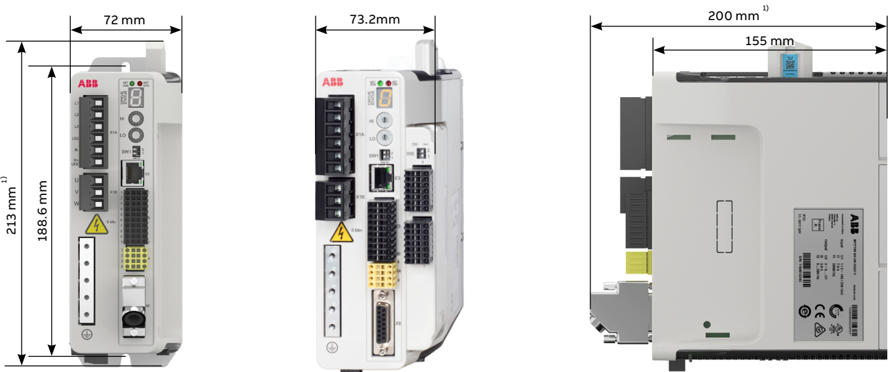
1) 近似尺寸。需为反馈和其它控制电缆留出额外空间。
